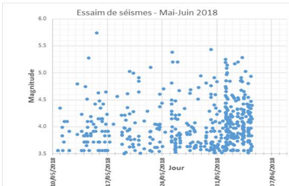
Suivi de l'essaim sismique en cours sur Mayotte : magnitudes des séismes en fonction du temps (en jour, à compter du 10/05/2018).
