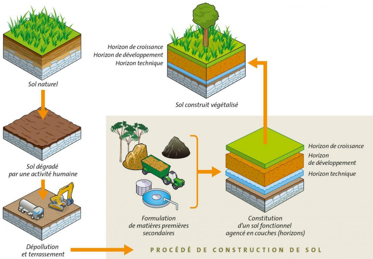
Schéma de synthèse illustrant l'intégration du procédé de construction de sol (Brevet INRA/INPL/TVD) pour la reconquête des milieux dégradés.
